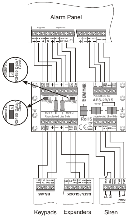
Ochrona 2 magistral i sygnalizatora bez własnego zasilania
